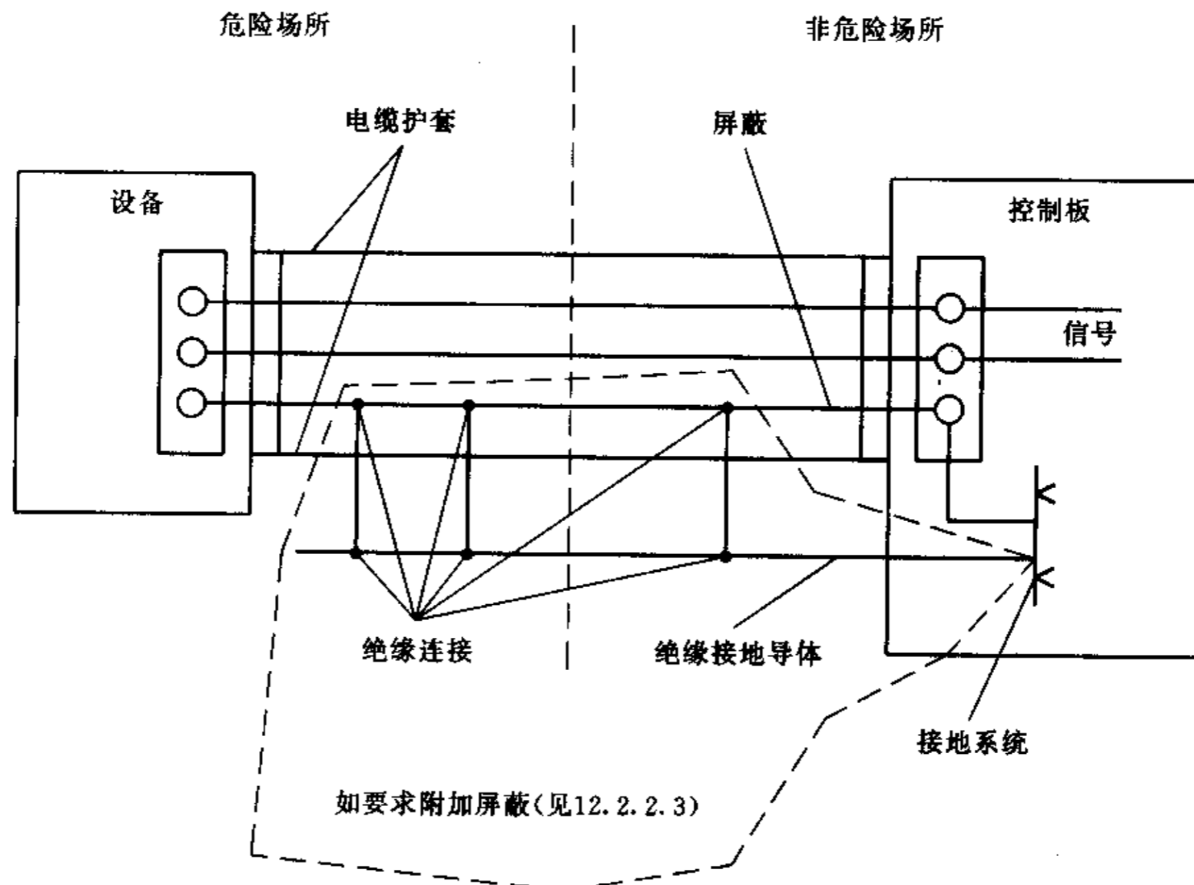
图2 导电屏蔽接地
